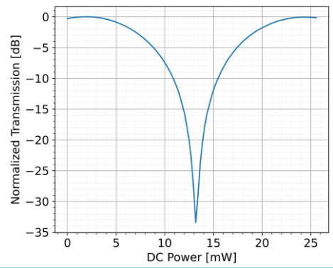
O/C band bMZM
